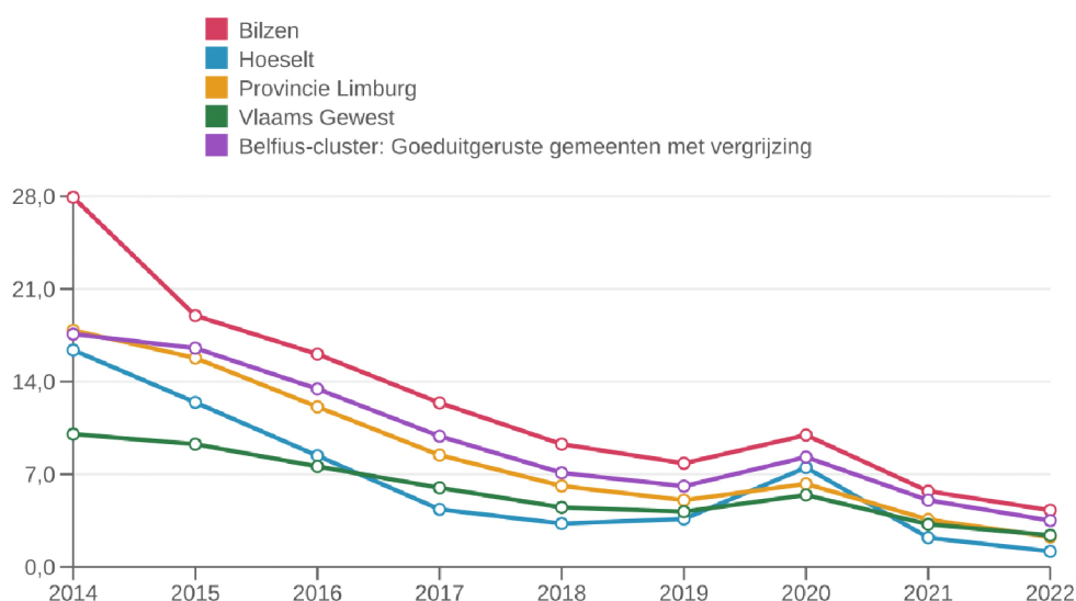
Spanningsratio, 2014-2022, verhouding
