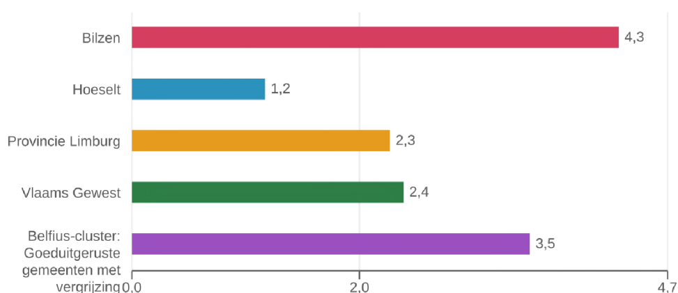
Spanningsratio, 2022, verhouding
